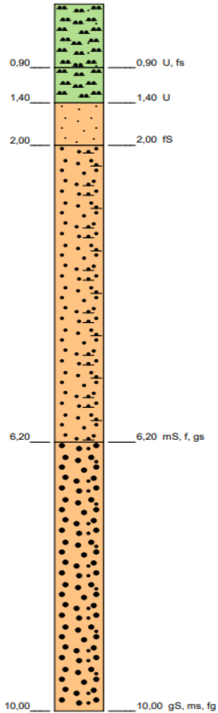
Abb. 1: Vorprofil GWM Neufriedland 1/26
